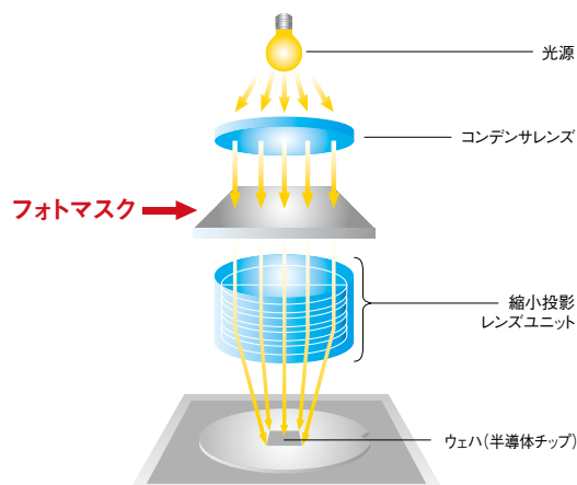
半導体製造の露光工程における回路パターン転写のイメージ
