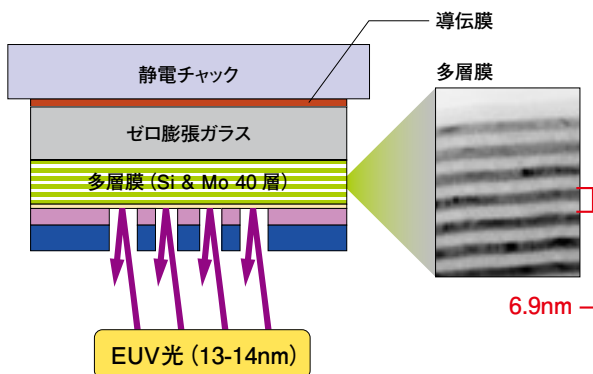
反射型EUVマスク(イメージ)
