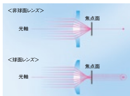
非球面モールドレンズと球面レンズの比較
